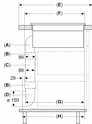
Mitat mm
