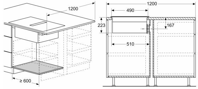
Mitat mm
