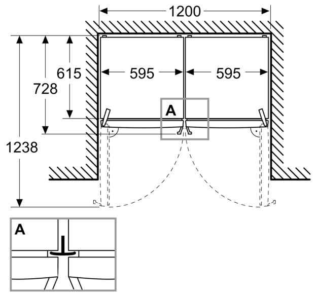
Mitat mm
