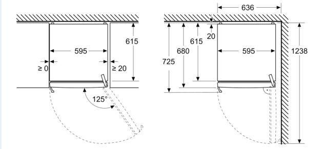
Mitat mm
